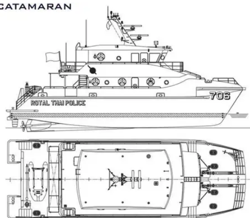
23M. CATAMARAN
